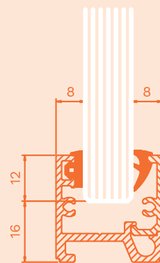
N28 med kilgummi 2, för 12-12,76 mm glas.
