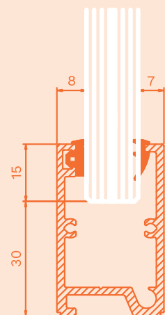
N45 med kilgummi 1, för 13,52 mm glas.
