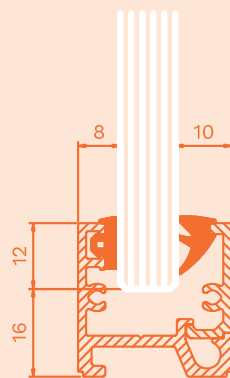
N28 med kilgummi 3, för 10-10,76 mm glas.
