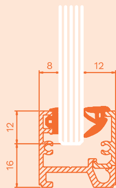
N28 med kilgummi 4, för 8-8,76 mm glas.
