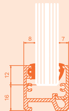
N28 med kilgummi 1, för 13,52 mm glas.
