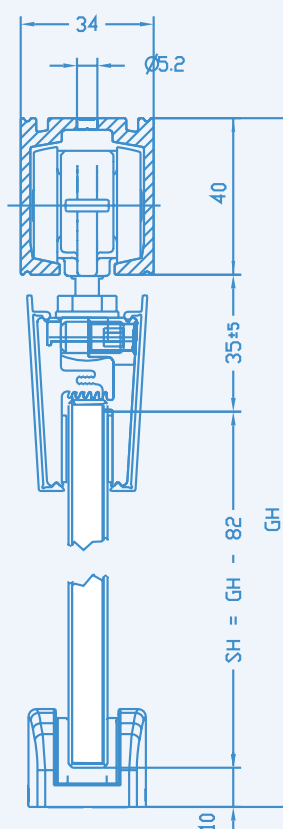
Mått Perlan 140, takmontage
