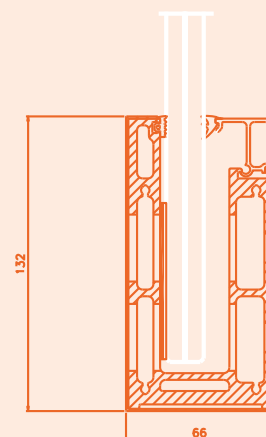
Sidomonterat med täckplåt
