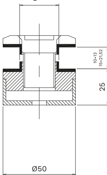
Borrhål i glas Ø30mm
